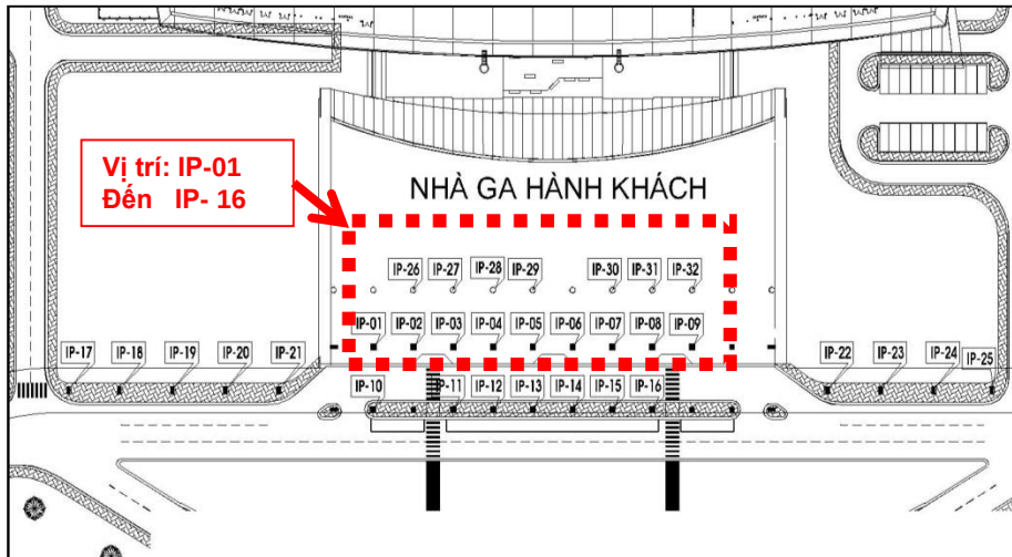
Mặt bằng vị trí hộp đèn ốp cột trụ cầu cạn
